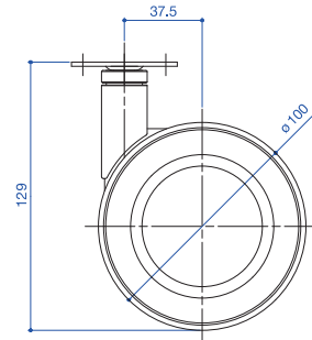
DE1-0EP-ZU2-100 平付けタイプ Plate stem type
